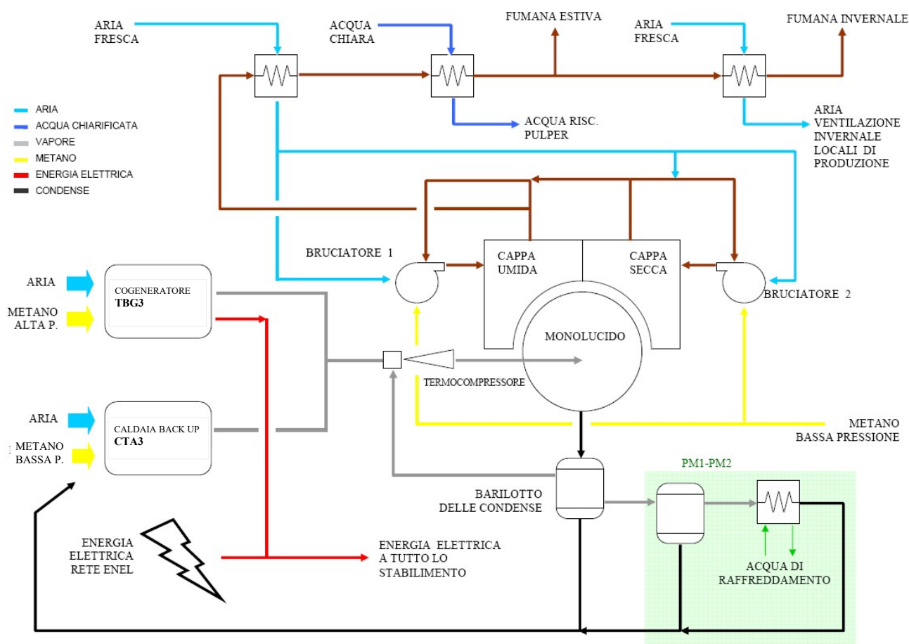
Fig. 8 Schema energetico di Soffass Via Lazzareschi
